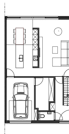
GELIJKVLOERS
