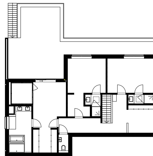
VERDIEPING
