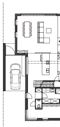
GELIJKVLOERS
