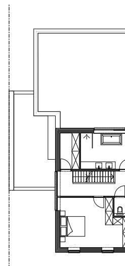
VERDIEPING
