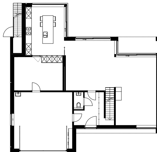
GELIJKVLOERS
