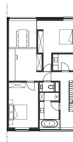
VERDIEPING
